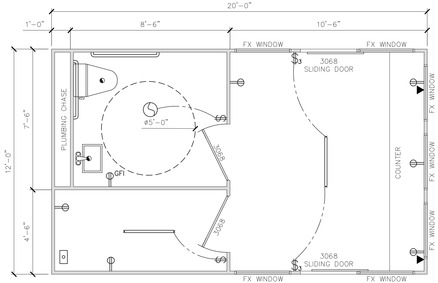
FLOOR PLAN SCALE: 3/8" = 1'-0"
